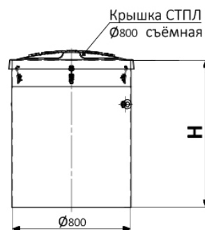
TK (A15) \varnothing 800
